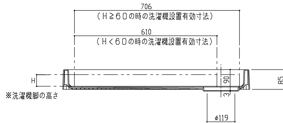
断面A-A
